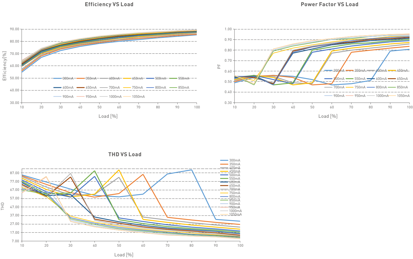
SE-40-300-1050-W1D
